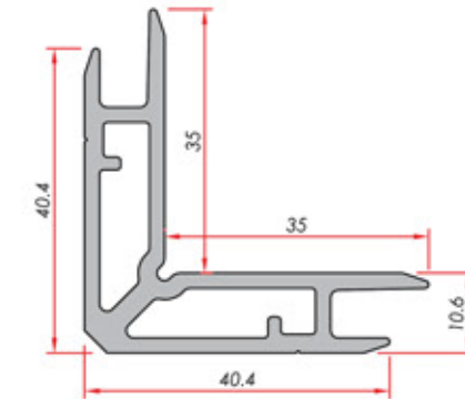
Corner Cleat Köşe Takoğu
