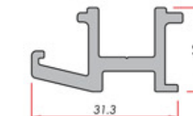
Panel Assembling Wedge Kaset Montaj Takozu
