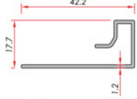
Dilatation Profile Dilatasyon Kapak
