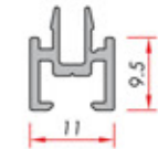
Single Glass Bead Tek Cam Çıtası
