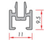
Single Glass Bead Tek Cam Çıtası
