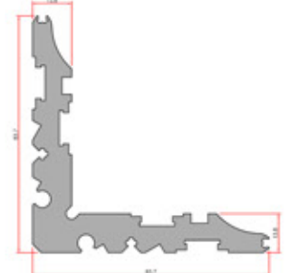
Corner Cleat Köşe Takozu
