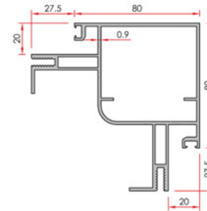
90° Corner Profile 90° Köşe Profili
