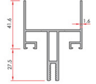
Mullion Profiles Mulyon Profilleri
