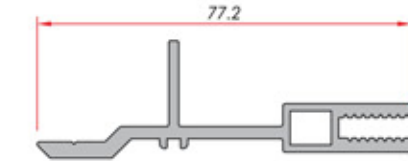
Half Mullion Adapter Yarım Mulyon Adaptörü
