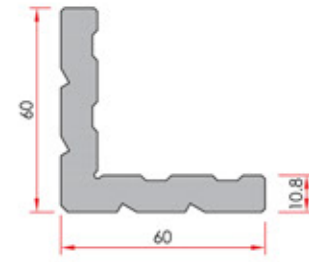
Corner Cleat Köşe Takozu
