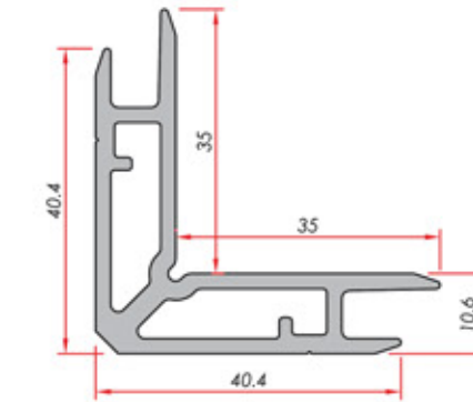
Corner Cleat Köşe Takozu
