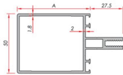
Transom Profiles Transom Profillerleri
