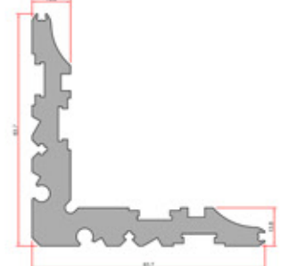
Corner Cleat Köşe Takozu
