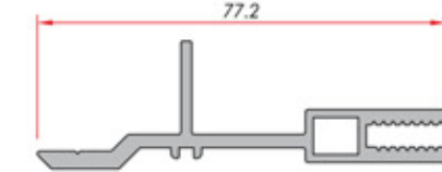
Half Mullion Adapter Yarım Mulyon Adaptörü
