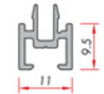
Single Glass Bead Tek Cam Çıtası
