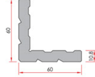
Corner Cleat Köşe Takozu
