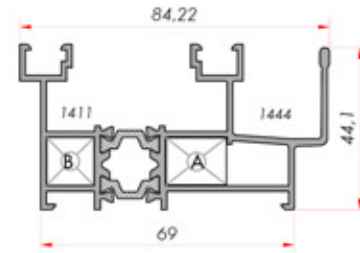
Mosquito Netting Rail Sineklik Raylı Kasa Profili
