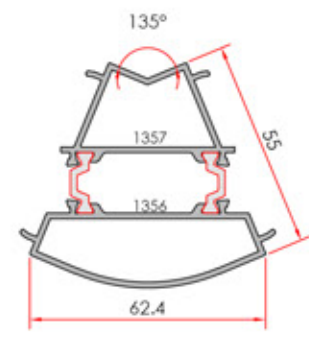
135° Corner Adapter 135° Köşe Dönüş Adaptörü
