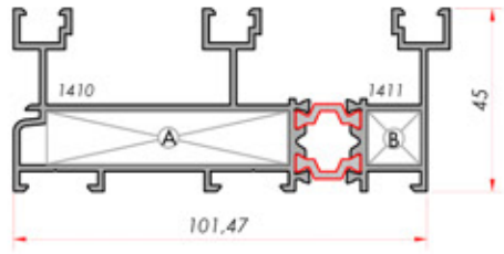
Three Rail Frame Üç Raylı Kasa
